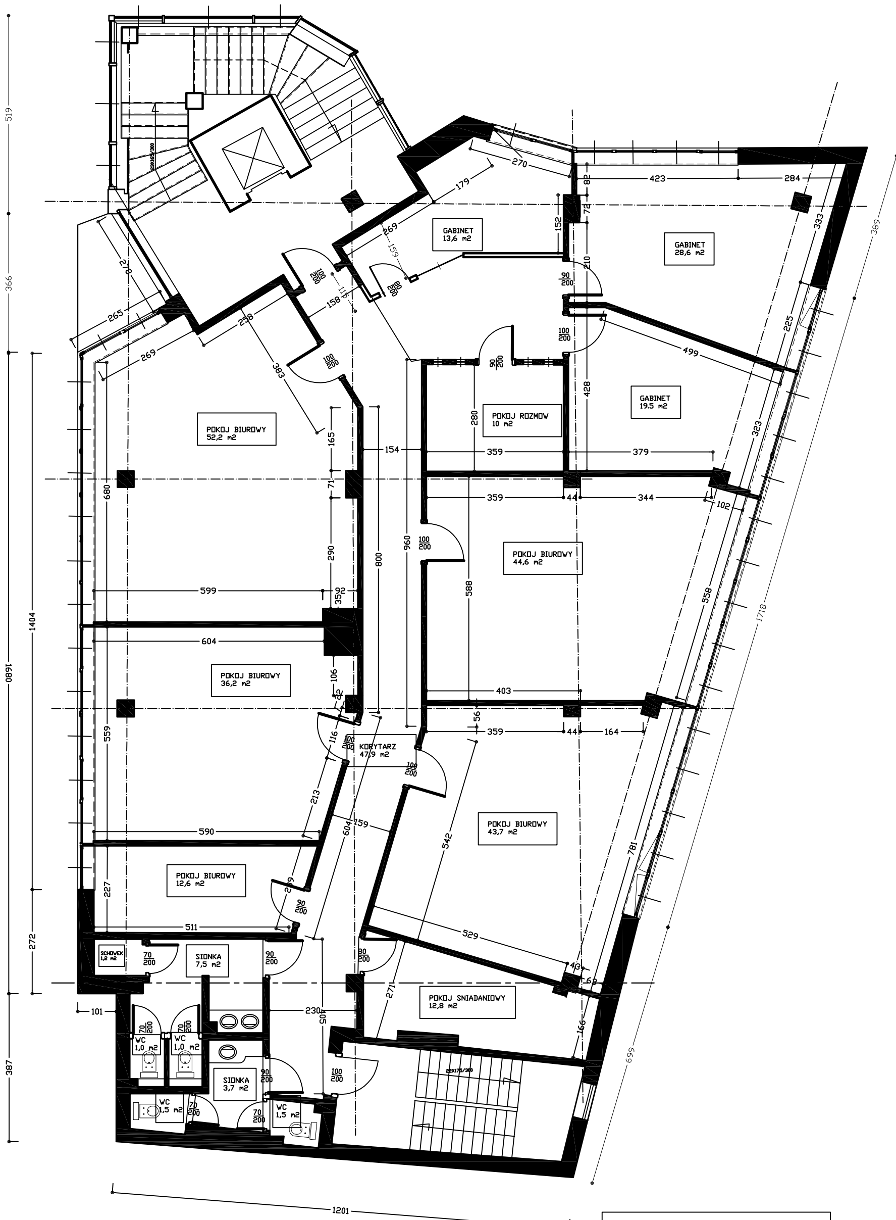
BUDYNEK BIUROWY Al. Krakowska rzut 1 pietra stan 04' 2013 skala 1-100
